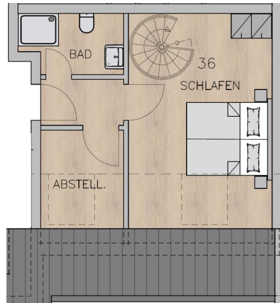
Dachgeschoss
